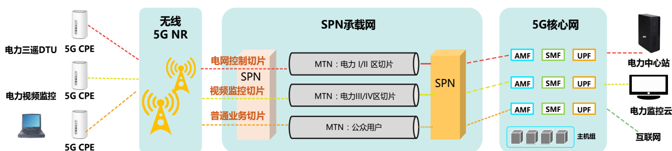
图7 电网切片组网
