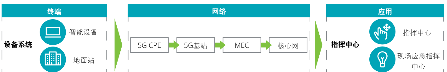
图8：5G智慧环保技术框架
