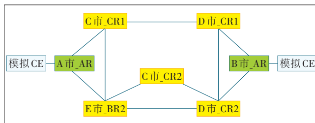
图2 现网试点组网拓扑
